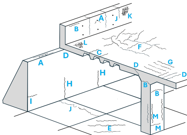
Figuur 1: Veel voorkomende scheurpatronen in beton
