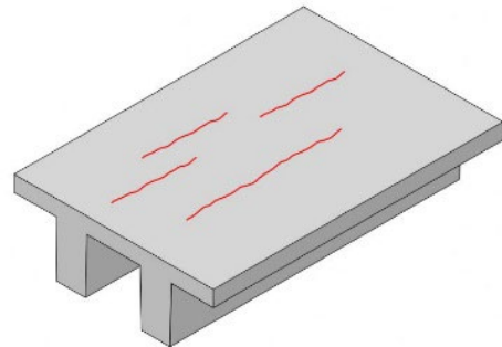
Figuur 3: Scheurvorming ter plaatse van veranderde hoogte (type C)
