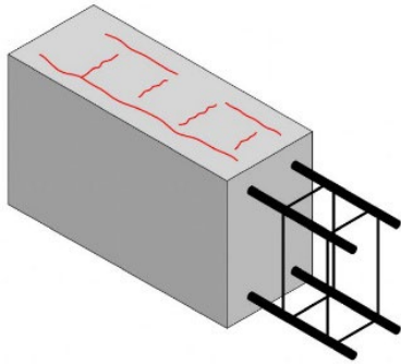
Figuur 2: Zettingscheuren ter plaatse van wapening, bovenzijde wand (type A)
